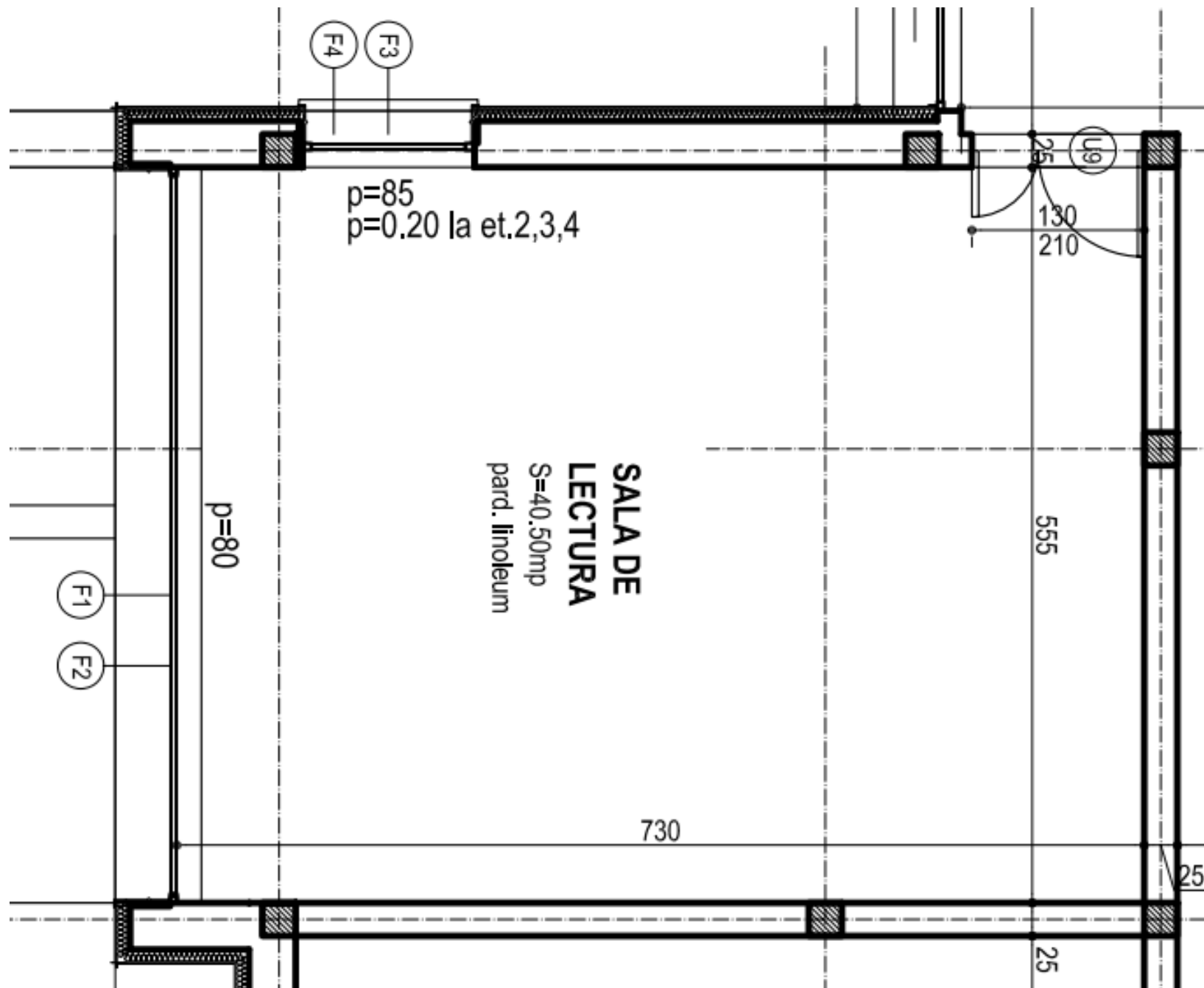
Plan aferent spațiilor din căminele T9, T10, T11
